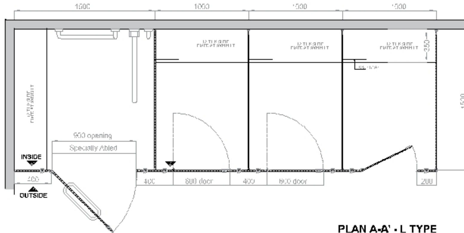
PLAN A-A' - L TYPE
