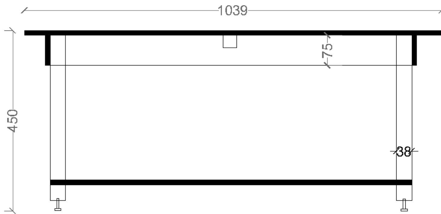
ELEVATION
