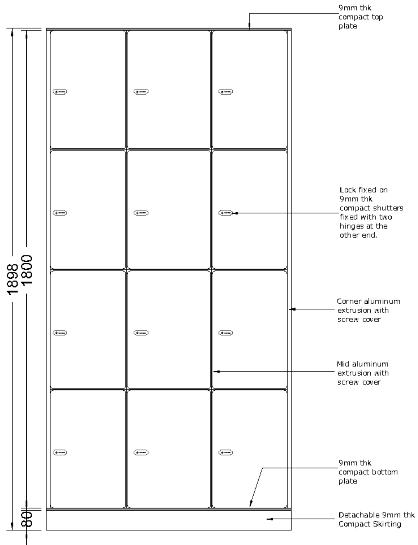
ELEVATION
